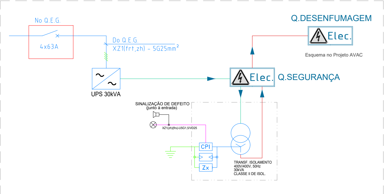
DIAGRAMA DA LIGAÇÃO DO QUADRO DE DESENFUMAGEM
